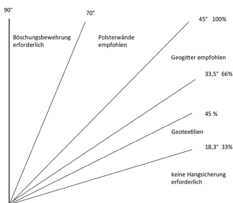
Abb.3.3: Böschungsneigung und Verfahren zur Hangsicherung (nach Zimmermann 2009)
